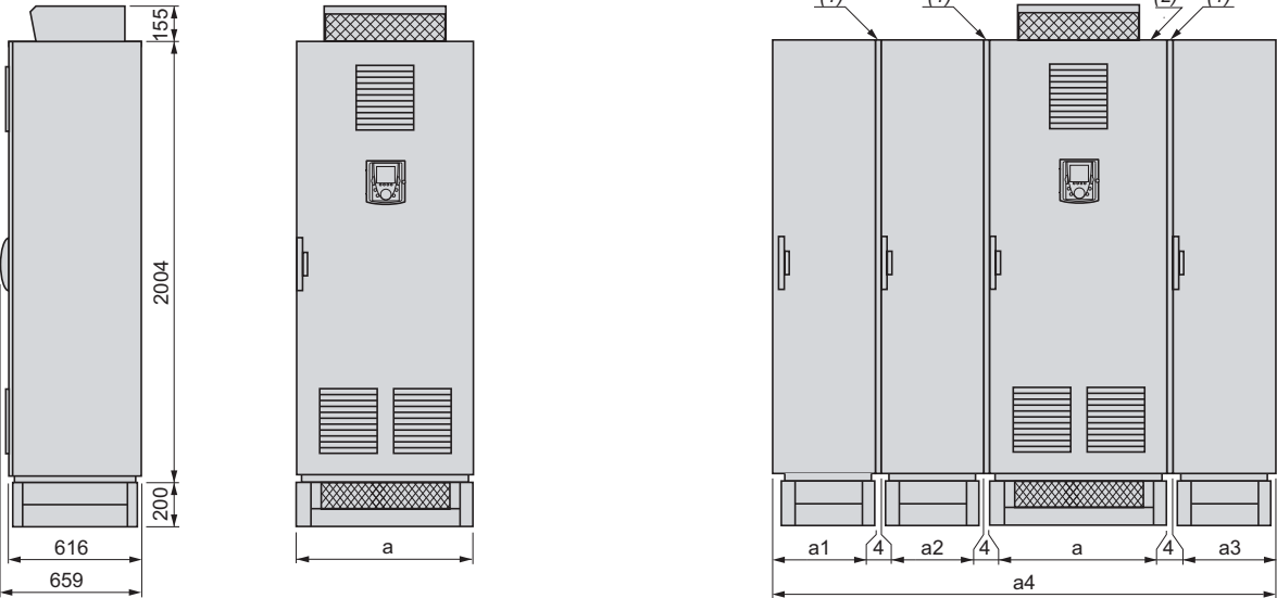
Комплектные ПЧ в шкафах IP 54 с отдельным охлаждением (продолжение) ATV 71 EXS5C31N4 - EXS5C50N4, ATV 71 EXS5C31N - EXS5C50N, ATV 71 EXS5C40Y - EXS5C63Y Общий вид шкафа Базовый шкаф Базовый шкаф + дополнительные шкафы в зависимости от конфигурации
