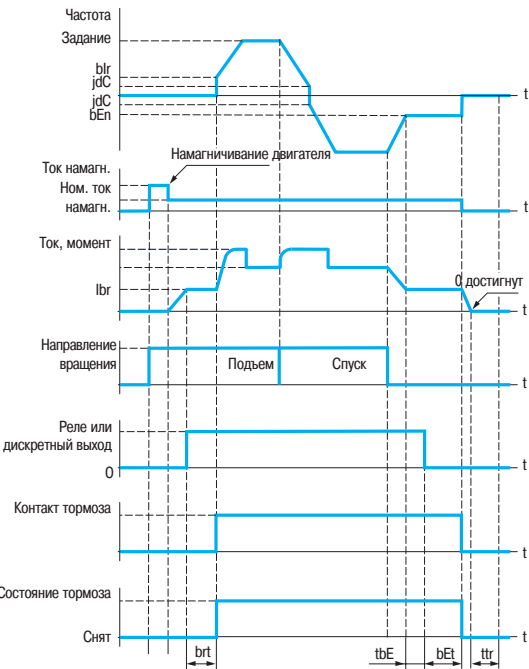
Вертикальное перемещение с разомкнутой системой управления
