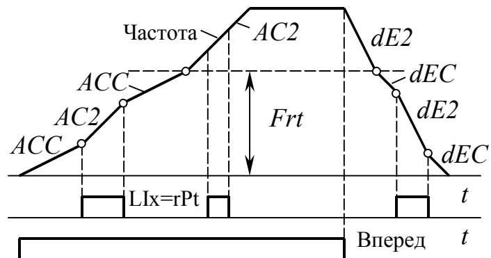
Рис. 9.9. Переключение темпов
