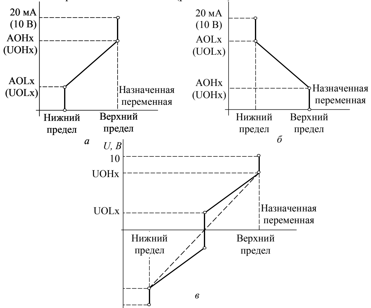
Рис. 7.11. Статические характеристики аналоговых выходов
