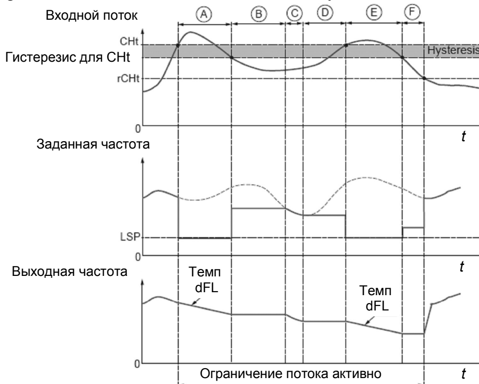
Рис. 9.14. Ограничение расхода
