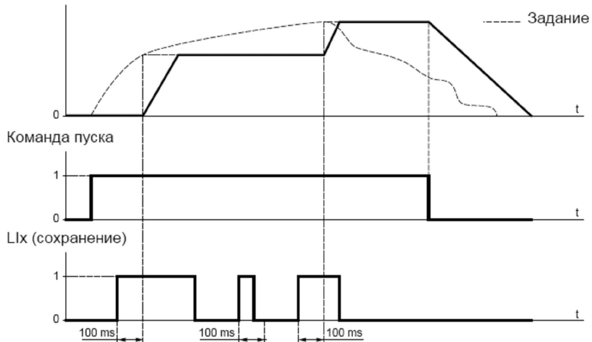
Рис. 9.5. Работа в режиме «Сохранение задания»
