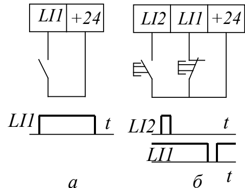
Рис. 7.2. Двухпроводное (а) и трехпроводное (б) управление
