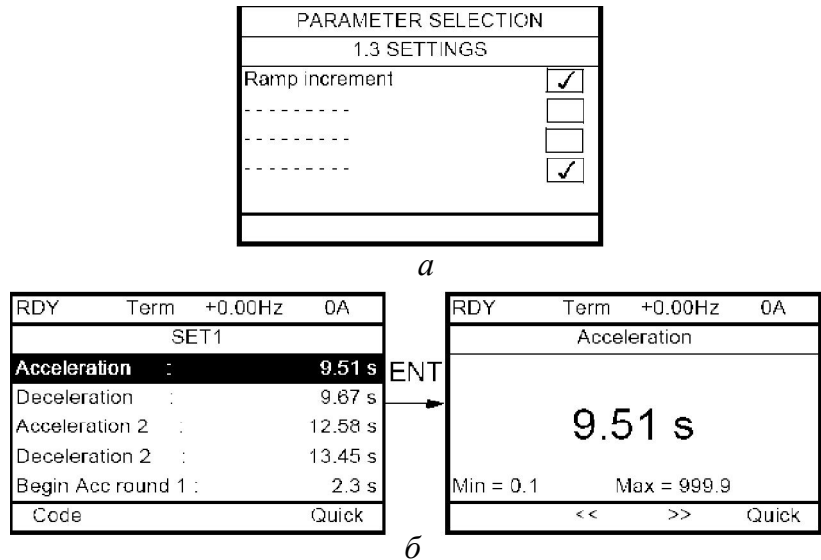
Рис. 9.8. Формирование комплекта параметров (а) и изменение их значений (б)
