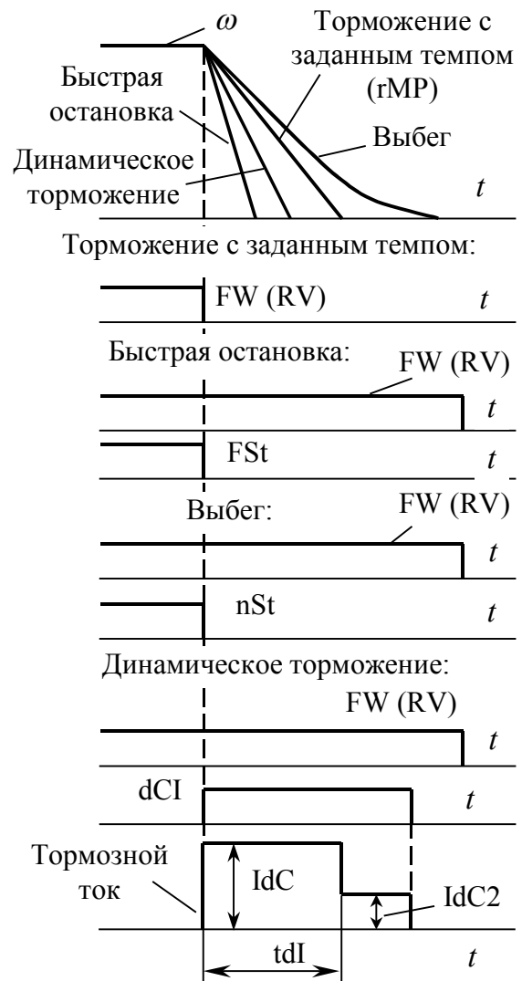
Рис. 5.4. Управление остановкой
