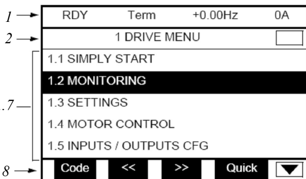
Рис. 1.2. Графический дисплей
