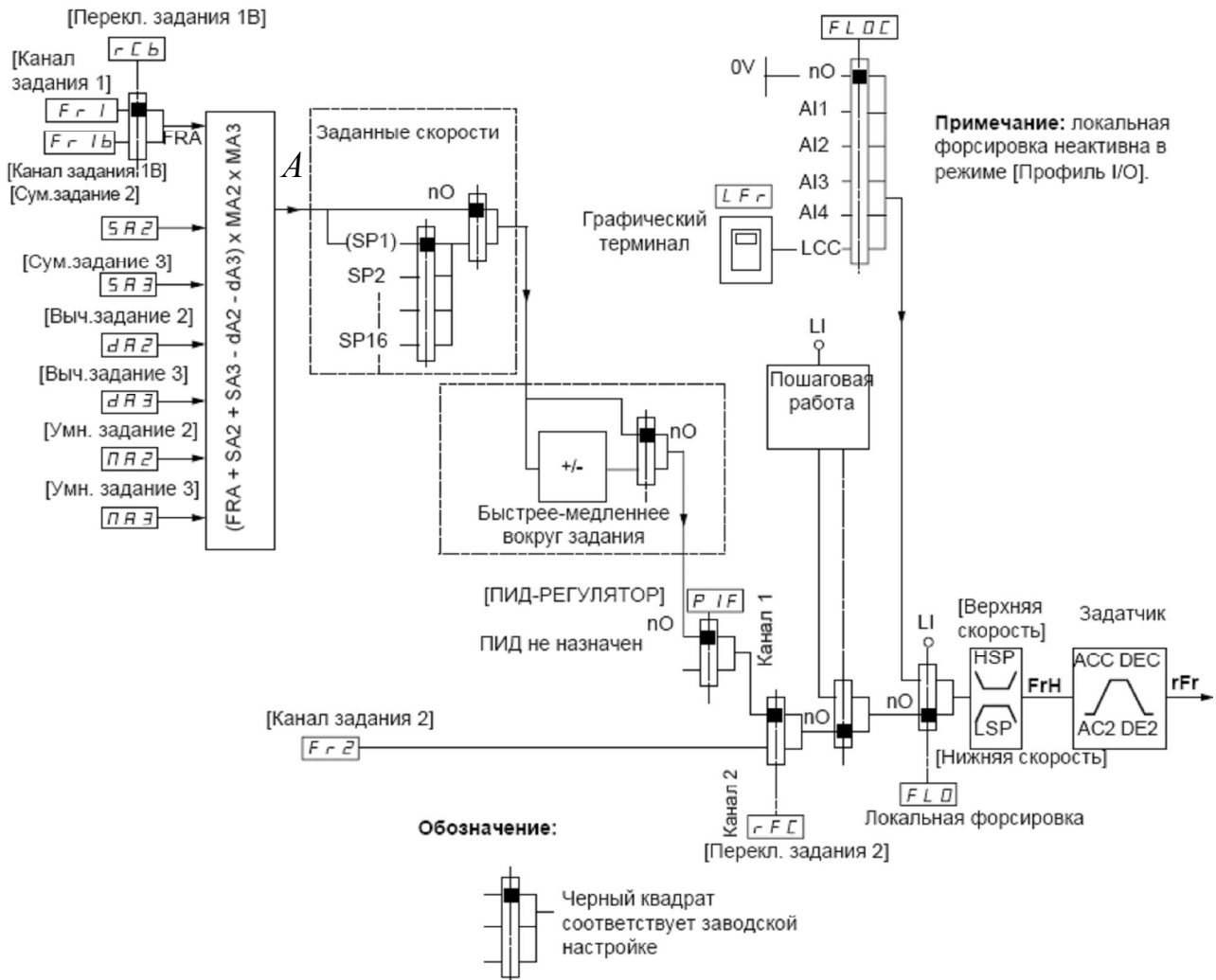
Рис. 8.2. Каналы задания при неконфигурированном ПИД-регуляторе
