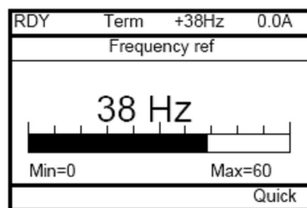
Рис. 1.5. Окно мониторинга
