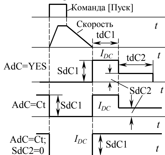
Рис. 5.5. Варианты удержания вала
