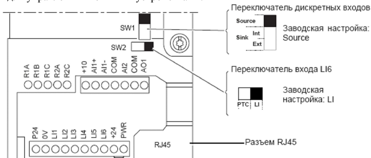
Рис. 7.1. Клеммы управления
