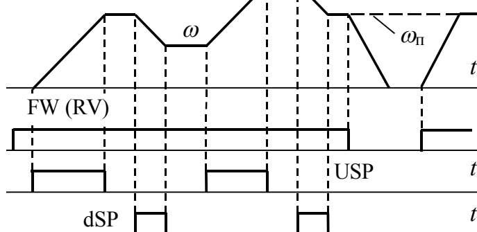
Рис. 9.3. Работа в режиме «быстрее-медленнее»
