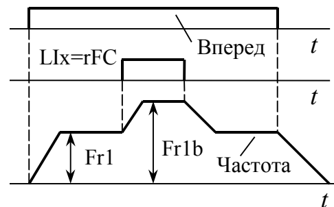
Рис. 8.1. Переключение заданий
