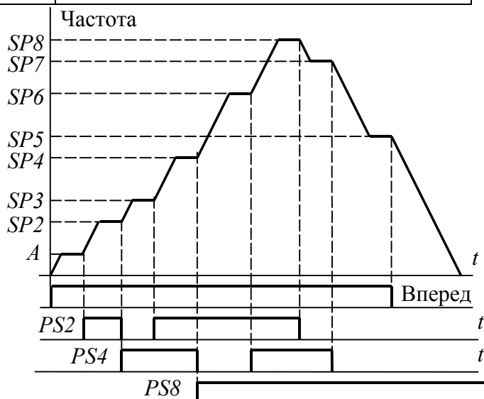
Рис. 9.2. Восьмиуровневая тахограмма
