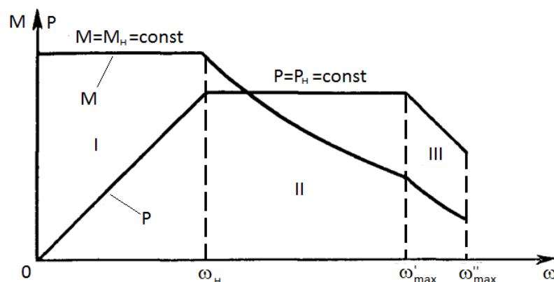
Рис. 1. Залежність максимальної потужності та обертального моменту від швидкості
