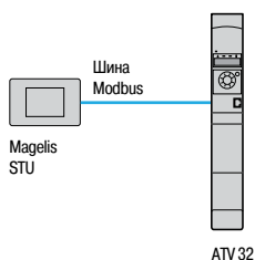
Пример конфигурации с использованием шины Modbus
