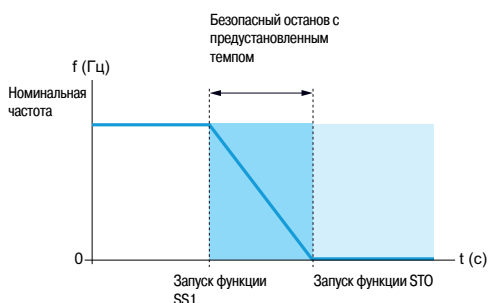
Запуск функции безопасности SS1
