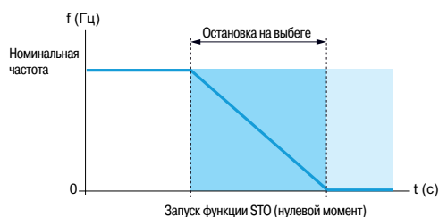
Запуск функции безопасности STO
