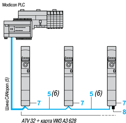
Пример подключения к шине CANopen с использованием клеммников с винтовыми зажимами
